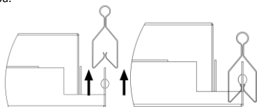
Рисунок 3 — Установка светильника Geniled серии Office Clip-In на подвесную конструкцию.
